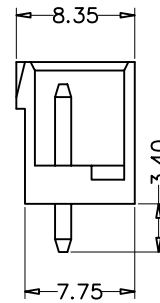
A-A SEC
